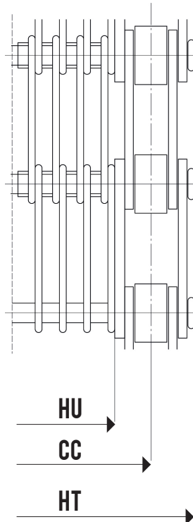
Tringles avec entretoises + chaînes latérales
